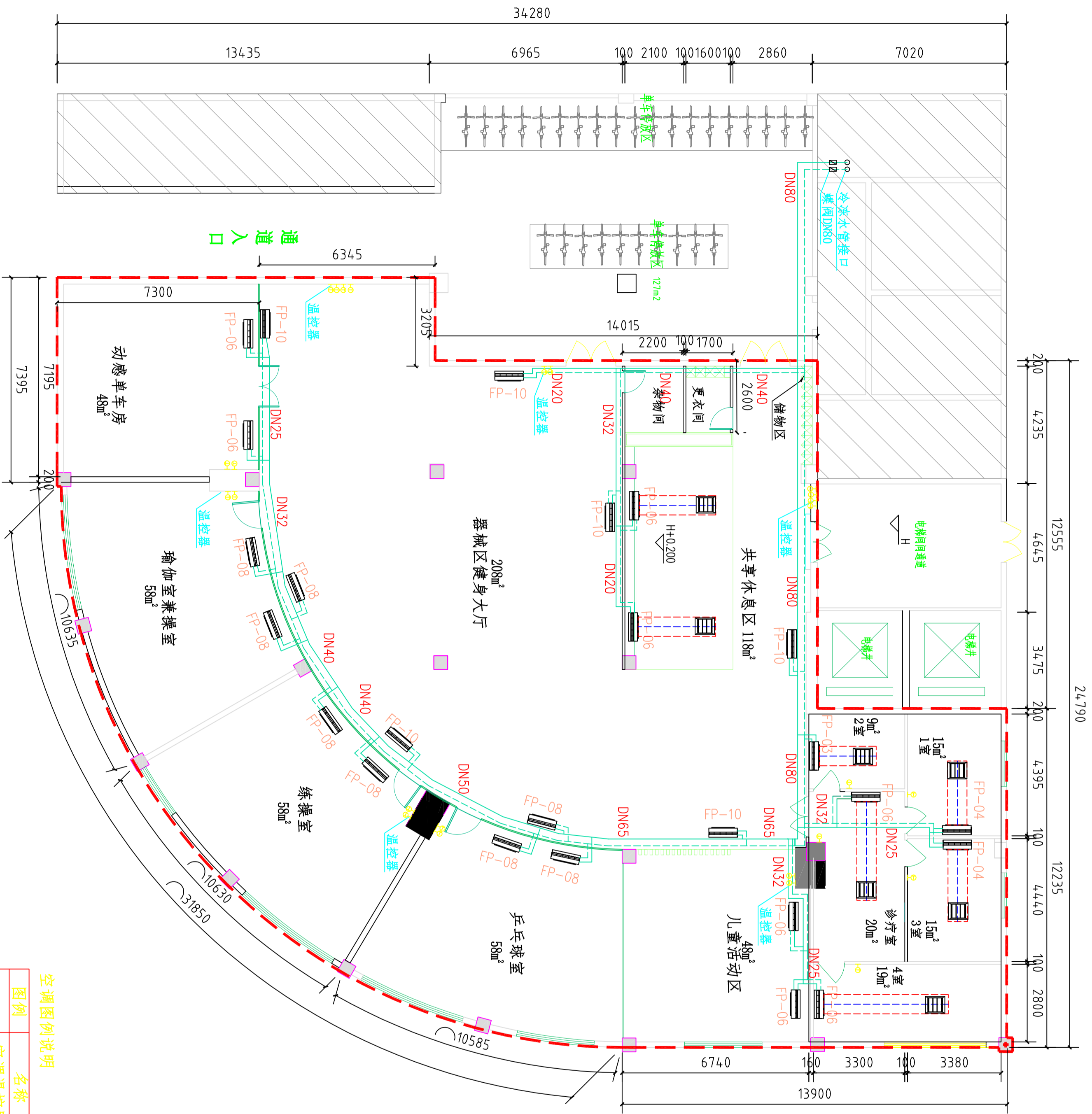
员工活动中心空调平面布局图 1:200
