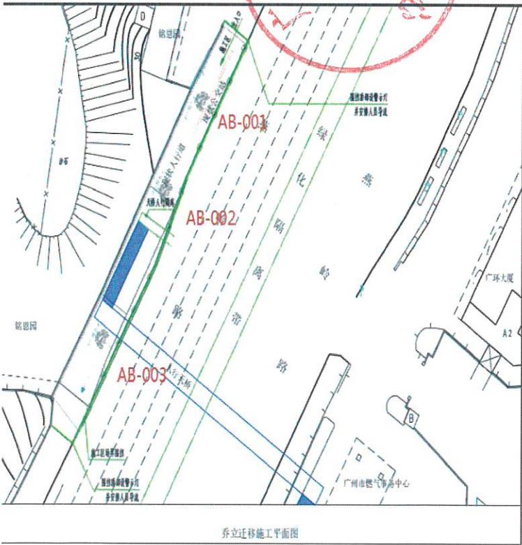
平面图
