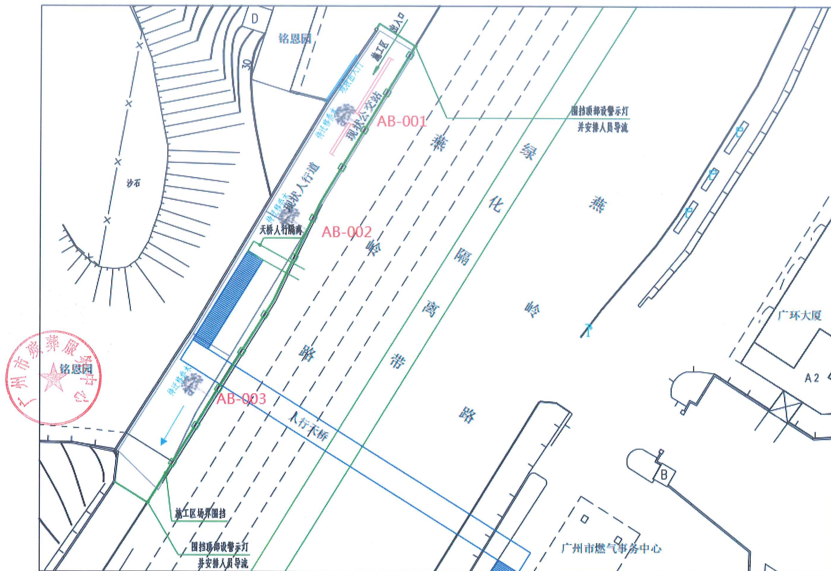
乔立迁移施工平面图
